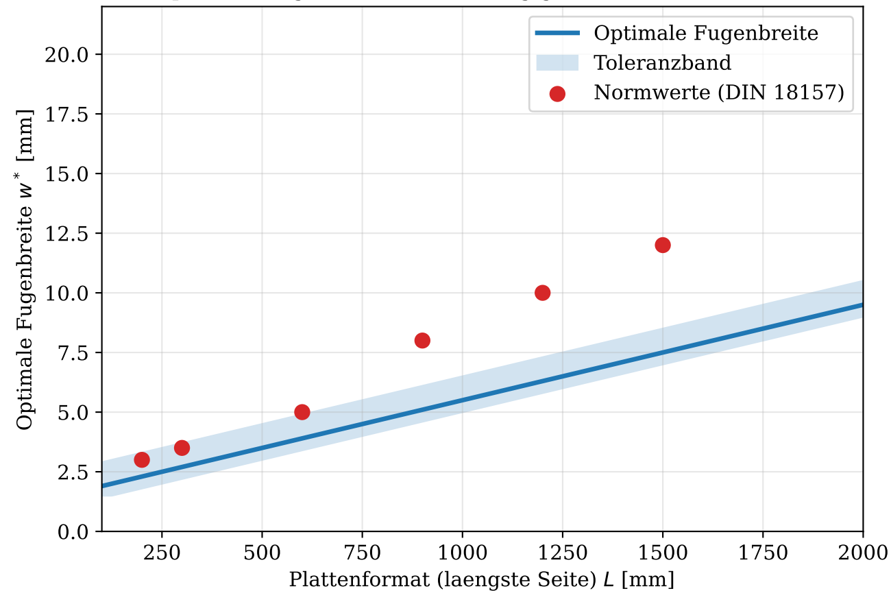
Optimale Fugenbreite in Abhängigkeit vom Plattenformat
