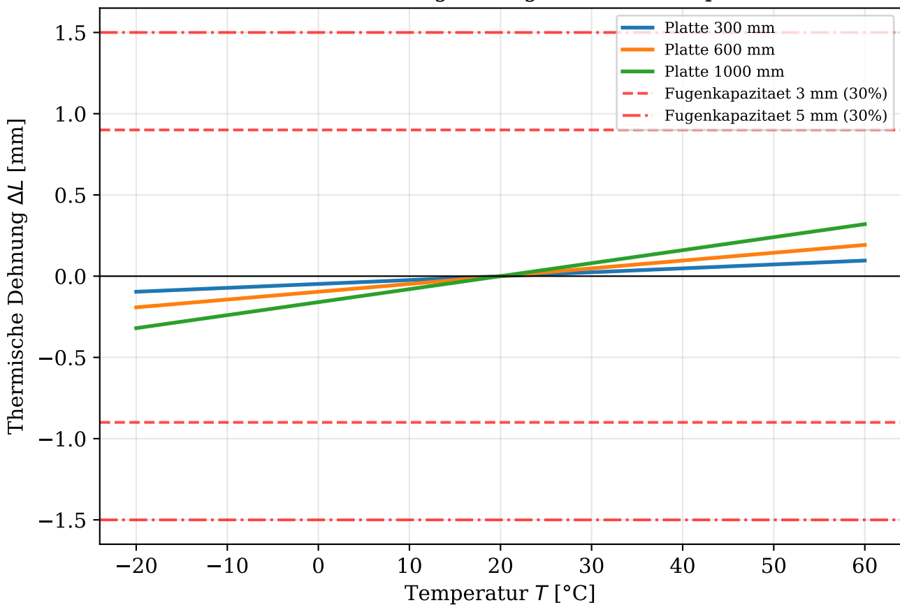
Thermische Dehnung vs. Fugenaufnahmekapazitaet
