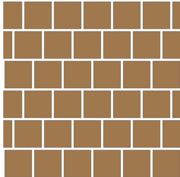
Drittelversatz (maximale Spannungsverteilung)
