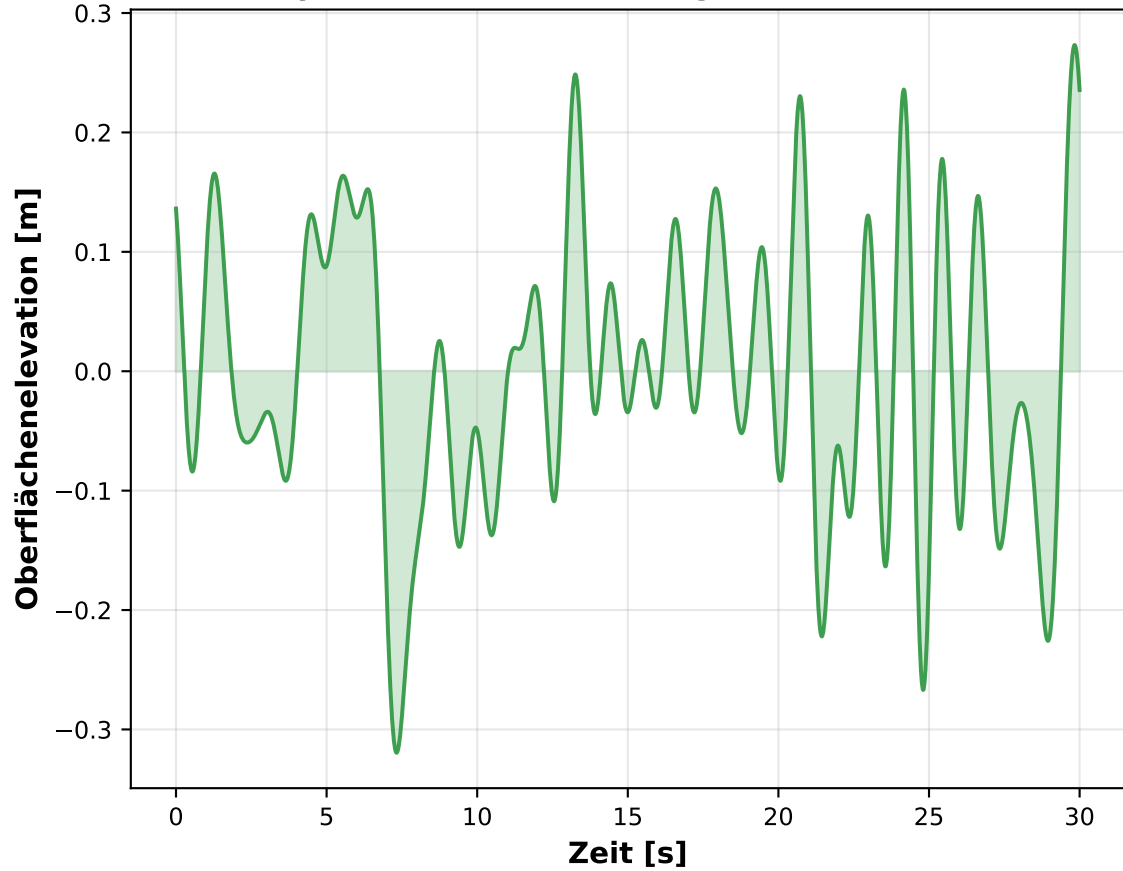
Synthetisches Wellensignal (JONSWAP)
