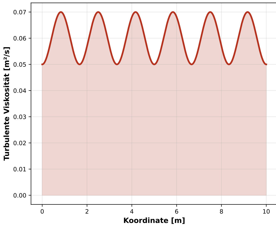
RANS: Turbulente Viskosität
