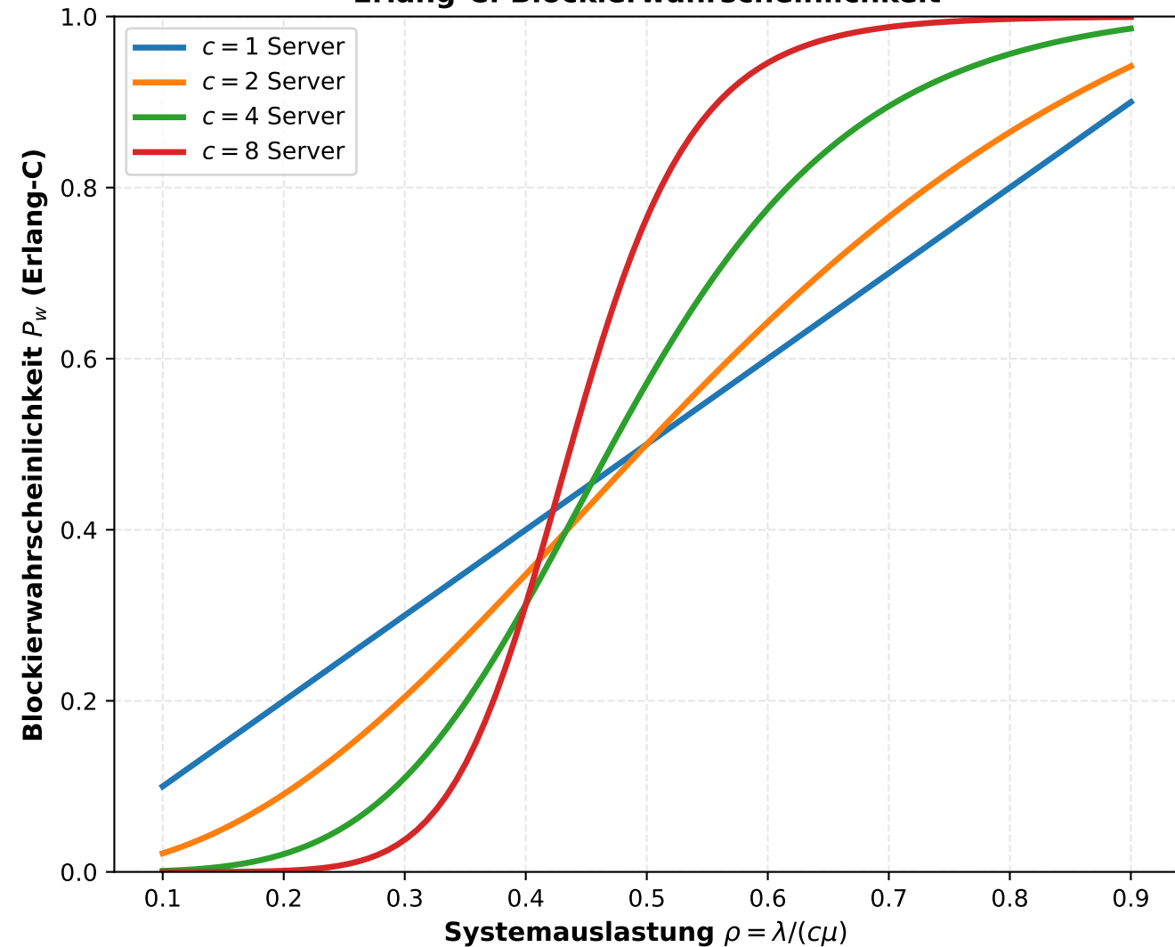
Erlang-C: Blockierwahrscheinlichkeit
