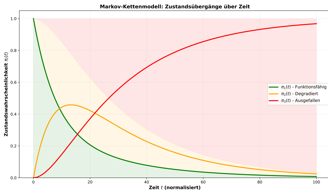
Figure 2: Markov-Kettenmodell mit 3 Zuständen: z_1 (Funktionsfähig, grün), z_2 (Degradert, orange), z_3 (Ausgefallen, rot). Zeigt die zeitliche Entwicklung der Zustandswahrscheinlichkeiten \pi_i(t) über eine Zeitspanne.
