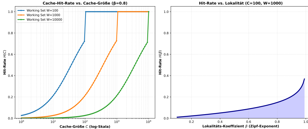
Figure 5: Cache-Hit-Rate unter Zipf-verteilten Zugriffen. Links: Hit-Rate vs. Cache-Größe für verschiedene Working Set Größen. Rechts: Hit-Rate vs. Lokaltäts-Koeffizient \beta .
