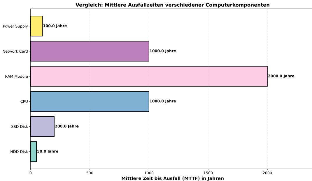
Figure 7: Mittlere Zeit bis Ausfall (MTTF) für verschiedene Computerkomponenten. Zeigt, daß mechanische Komponenten (HDDs, Power Supply) typischerweise viel früher ausfallen als elektronische Komponenten (CPU, RAM).
