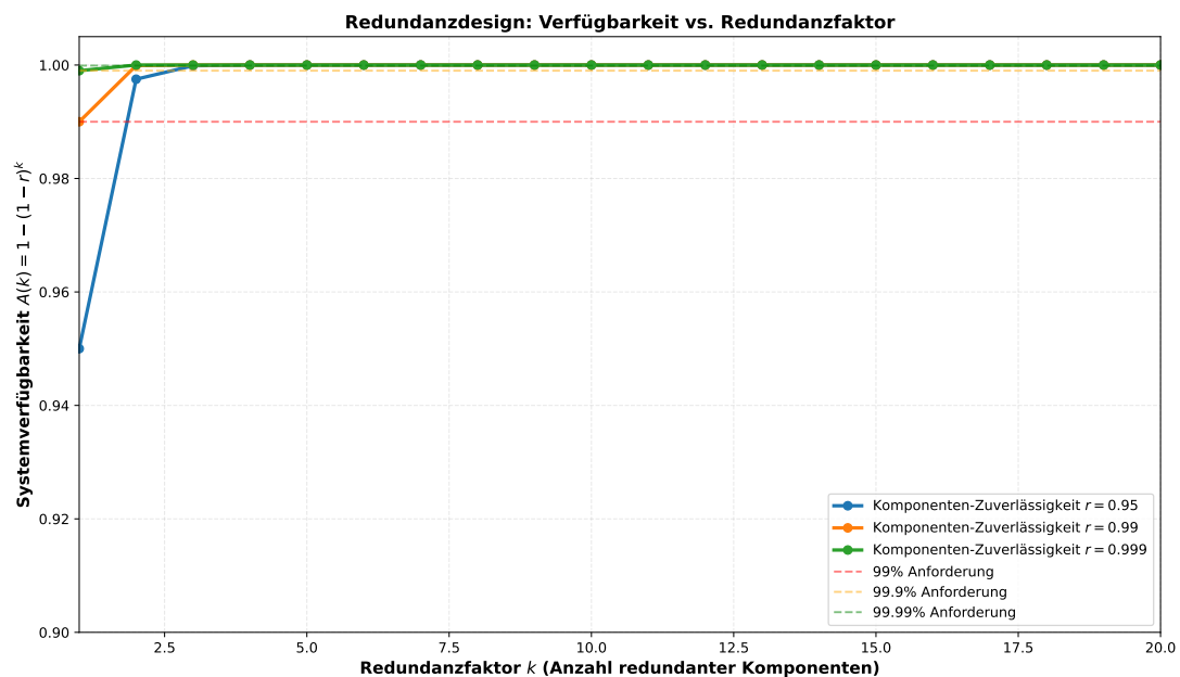
Figure 6: Redundanzdesign: Systemverfügbarkeit A(k) = 1 - (1 - r)^k vs. Redundanzfaktor k . Zeigt den Effekt von Redundanz auf die Verfügbarkeit für verschiedene Komponenten-Zuverlässigkeiten r .
