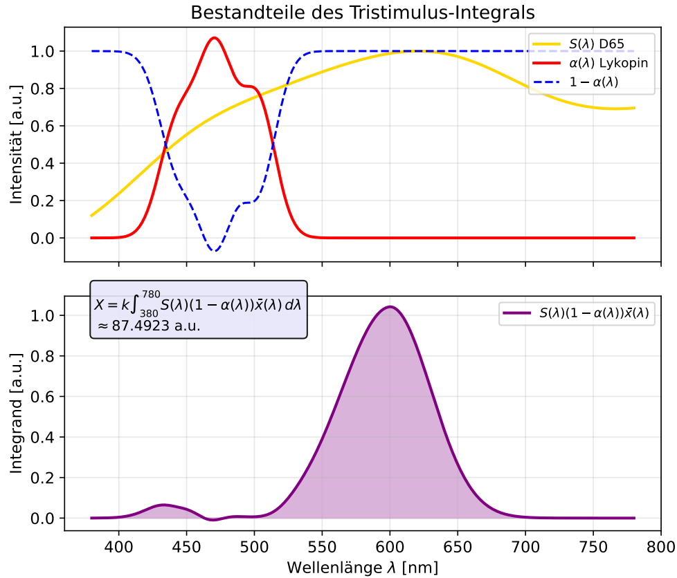
Figure 6: Oben: Spektrale Bestandteile des Tristimulus-Integrals für Lykopen unter D65: S(\lambda) (gold), \alpha(\lambda) (rot), 1 - \alpha(\lambda) (blau gestrichelt). Unten: Integrand S(\lambda)(1 - \alpha(\lambda))\bar{x}(\lambda) (lila) mit gefülltem Bereich. Das integrierte Ergebnis X ist eingeblendet.
