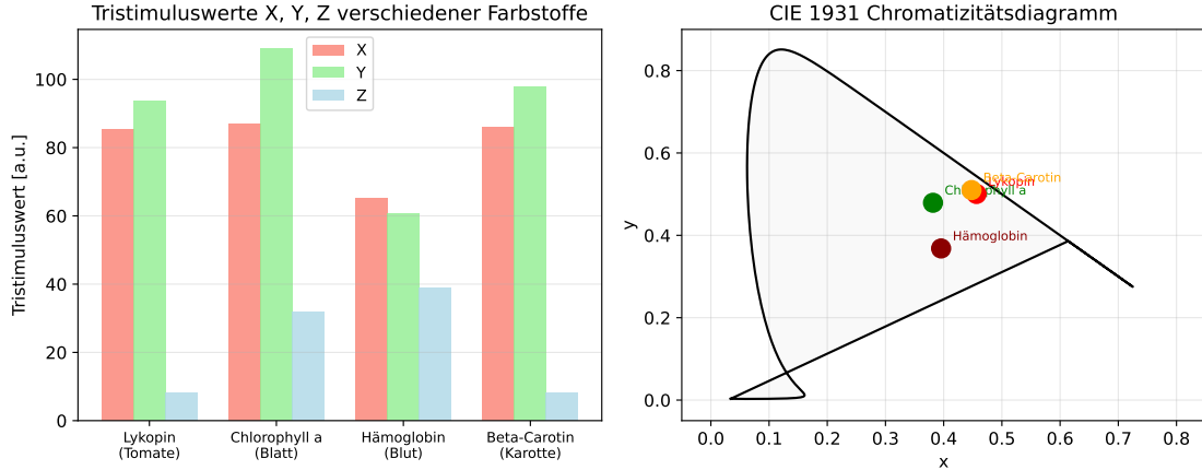
Figure 7: Links: Tristimuluswerte X, Y, Z für vier biologische Farbstoffe (Lykopen, Chlorophyll a, Hämoglobin, \beta -Carotin) unter D65-Beleuchtung. Rechts: Chromatizitätsdiagramm mit eingetragenen Farborten der Farbstoffe und der spektralen Linie (Hufeisenkurve).
