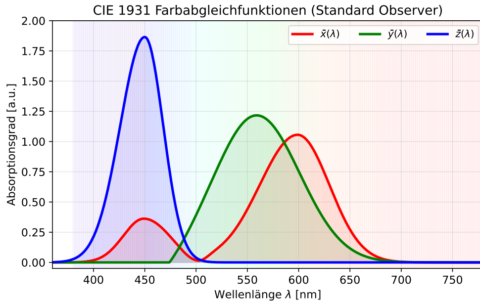
Figure 5: CIE 1931 Farbabgleichfunktionen \bar{x}(\lambda) (rot), \bar{y}(\lambda) (grün) und \bar{z}(\lambda) (blau) gemäß der Wyman-Näherung. Der gefärbte Hintergrund zeigt das sichtbare Spektrum. Die \bar{y}(\lambda) -Funktion entspricht der photopischen Hellempfindlichkeitskurve V(\lambda) .
