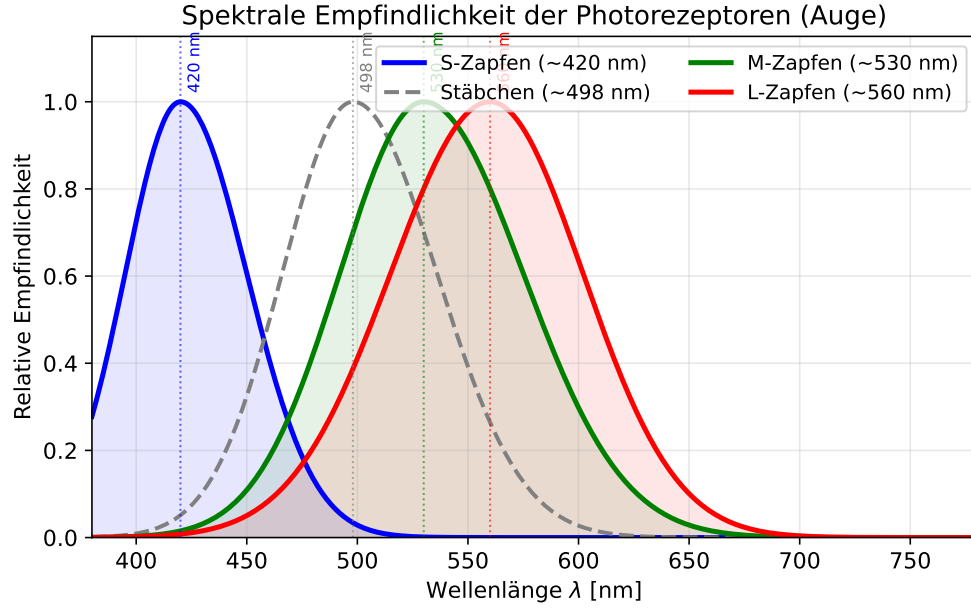
Figure 4: Spektrale Empfindlichkeiten der vier retinalen Photorezeptoren. Die Stäbchen (grau, gestrichelt) dominieren im Dämmerungssehen, die drei Zapfentypen (S: blau, M: grün, L: rot) ermöglichen das trichromatische Farbsehen am Tag.
