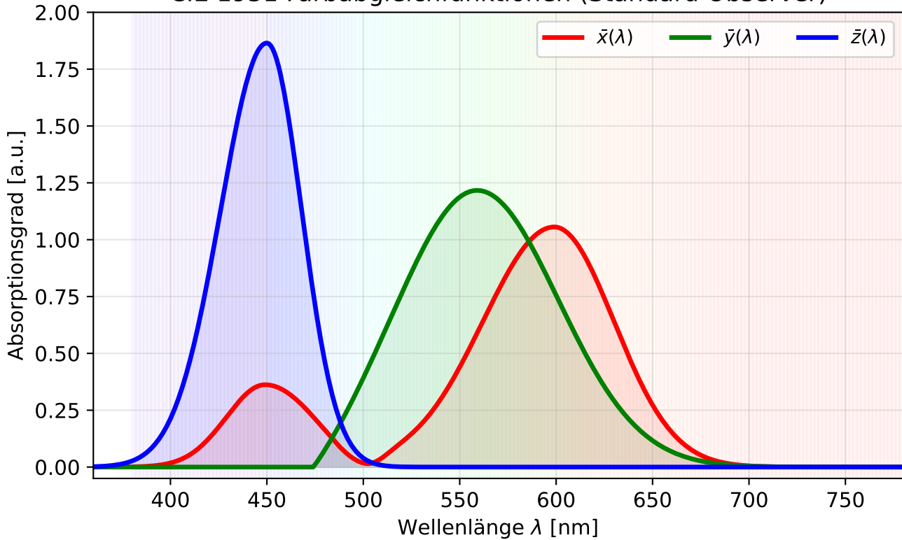
CIE 1931 Farbabgleichfunktionen (Standard Observer)
