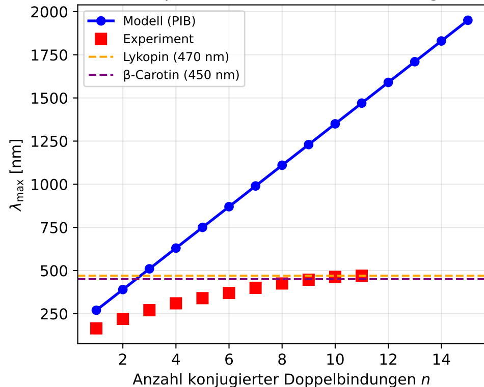
Absorptionsmaximum vs. Kettenlänge
