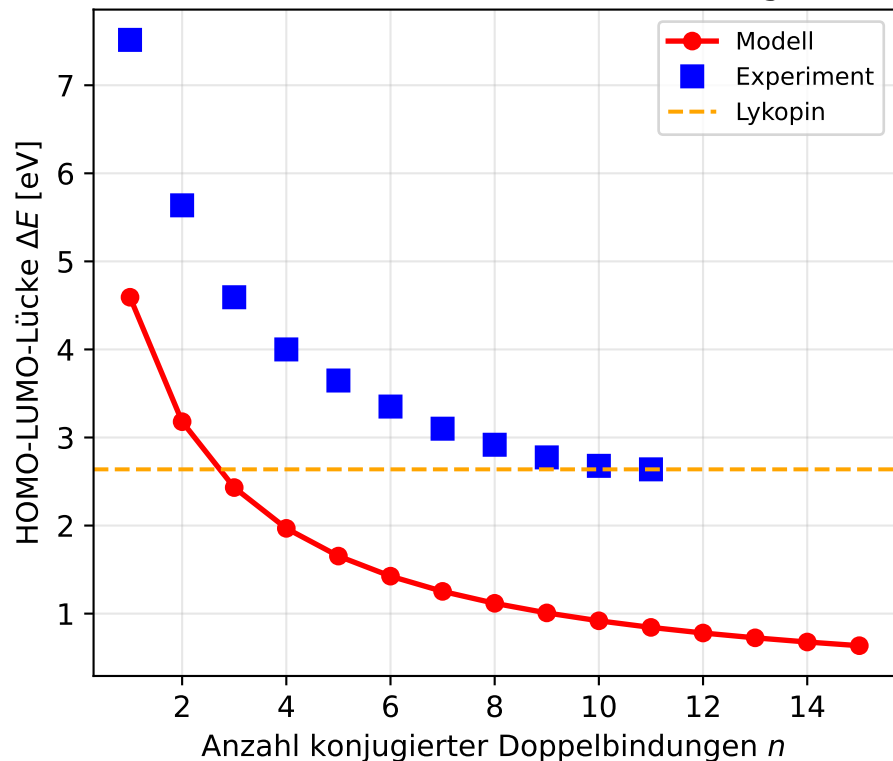
HOMO-LUMO-Lücke vs. Kettenlänge
