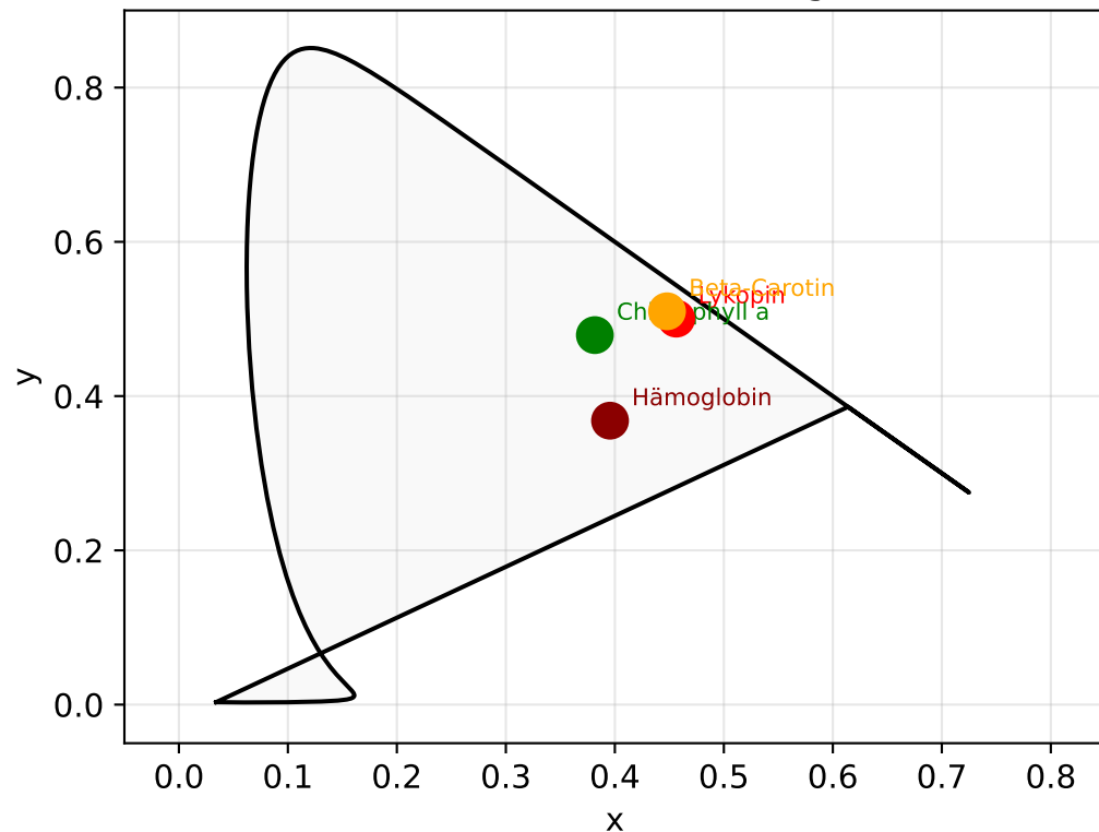
CIE 1931 Chromatizitätsdiagramm
