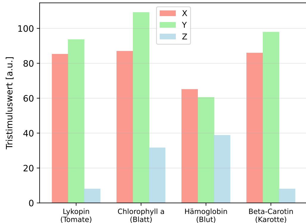
Tristimuluswerte X, Y, Z verschiedener Farbstoffe
