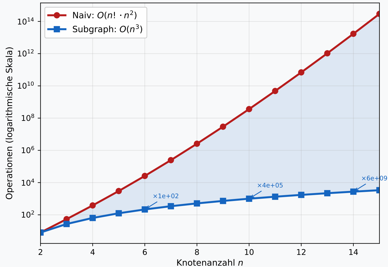
Laufzeitvergleich: Naiv vs. Subgraph (logarithmische Skala)
