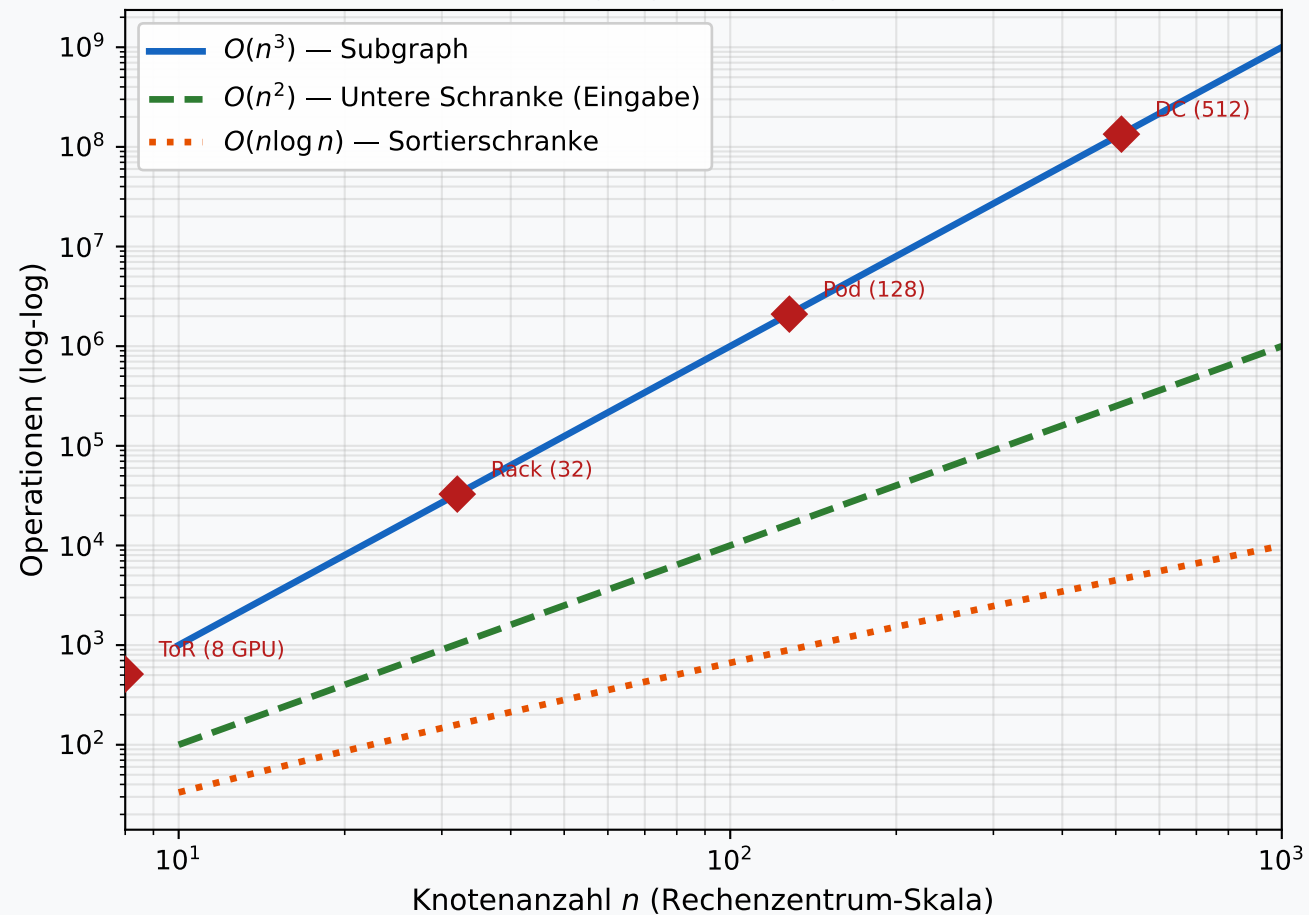
Komplexitätskurven — Rechenzentrum-Skalen (log-log Darstellung)
