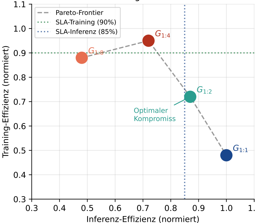
Pareto-Frontier: Inferenz vs. Training-Effizienz
