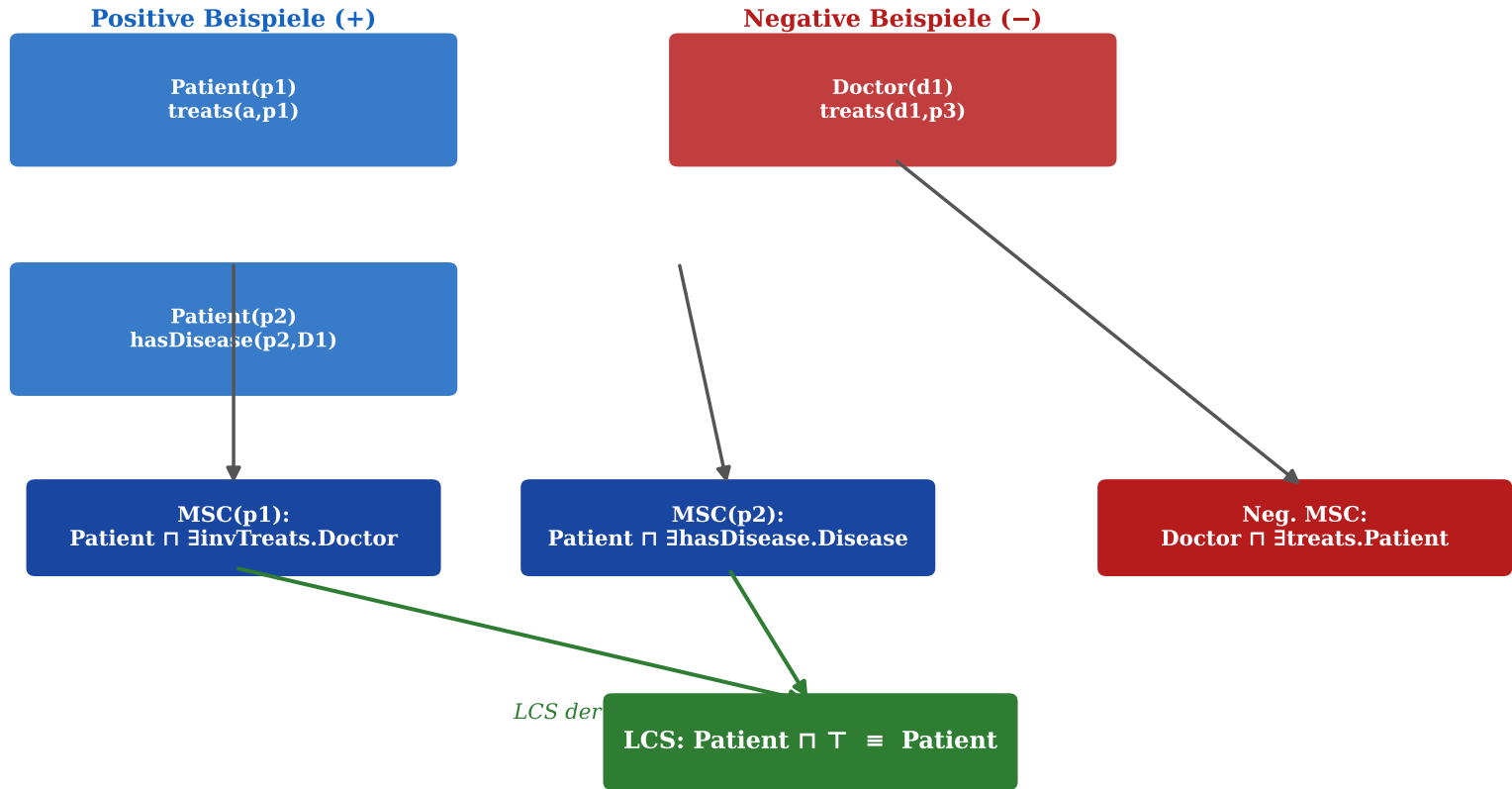
Abbildung 5: Lernen von DL-Konzepten mittels MSC und LCS
