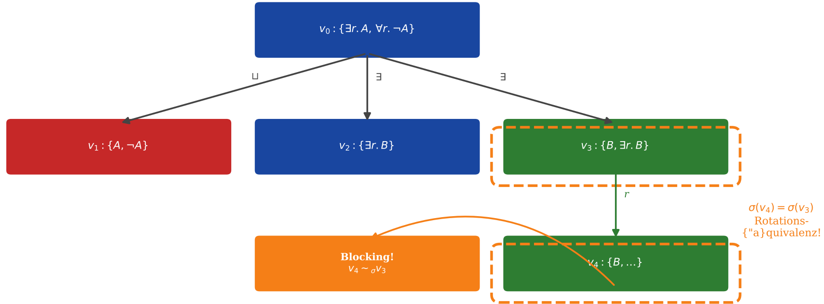
Abbildung 9: Tableau-Ast als gerichteter Graph -- Blocking \equiv Subgraph-Rotations{"a"}quivalenz
