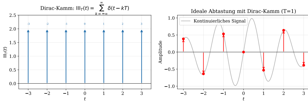
Figure 6: Links: der Dirac-Kamm \text{III}_T mit T = 1 , eine unendliche Folge äquidistanter Dirac-Impulse. Rechts: ideale Abtastung eines kontinuierlichen Signals durch Multiplikation mit dem Dirac-Kamm – die roten Pfeile repräsentieren die Abtastwerte.
