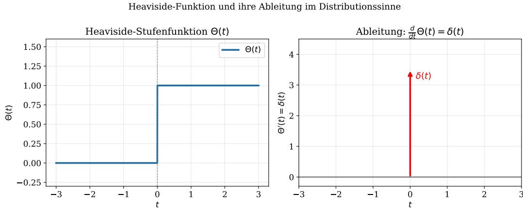
Figure 3: Links: die Heaviside-Stufenfunktion \Theta(t) . Rechts: ihre Ableitung im Distributionensinne ist der Dirac-Impuls \delta(t) . Der vertikale Sprung der Stufenfunktion um 1 entspricht formal der unendlichen Konzentration.
