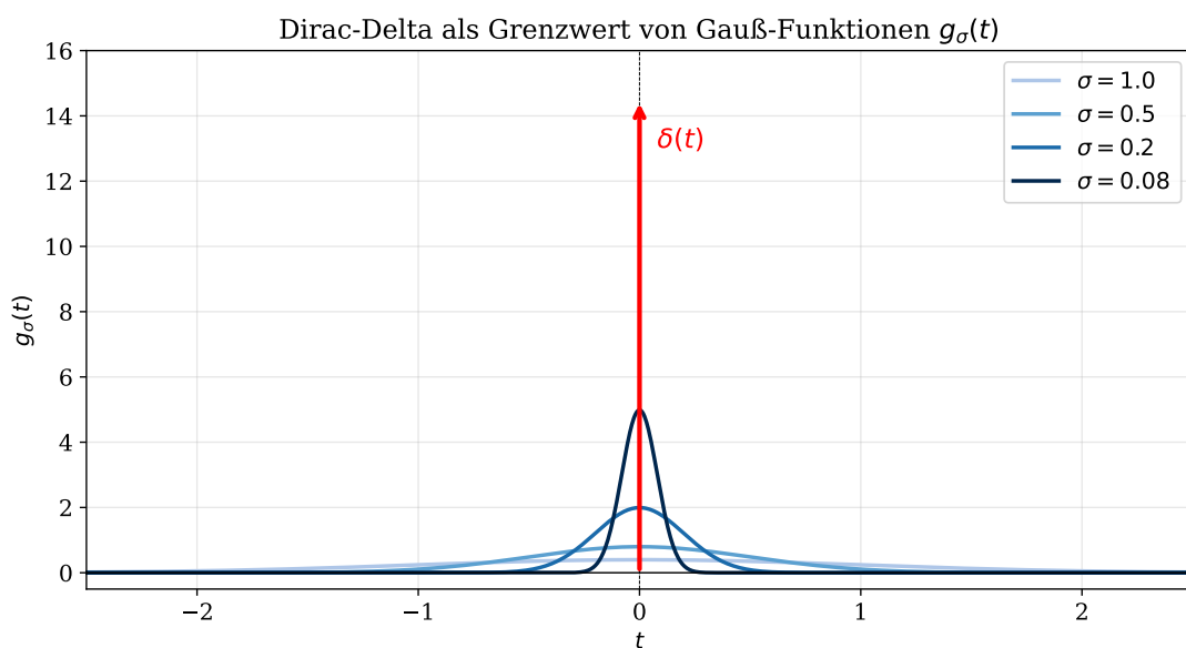
Figure 1: Der Dirac-Impuls als Grenzwert der Gaußschen Näherungsfolge g_{\varepsilon}(t) = \frac{1}{\varepsilon\sqrt{2\pi}} \exp(-t^2/(2\varepsilon^2)) . Mit kleiner werdendem \varepsilon wird die Spitze bei t = 0 beliebig hoch, während die Fläche stets gleich 1 bleibt. Der rote Pfeil symbolisiert den Grenzwert \delta(t) im Distributionensinne.
