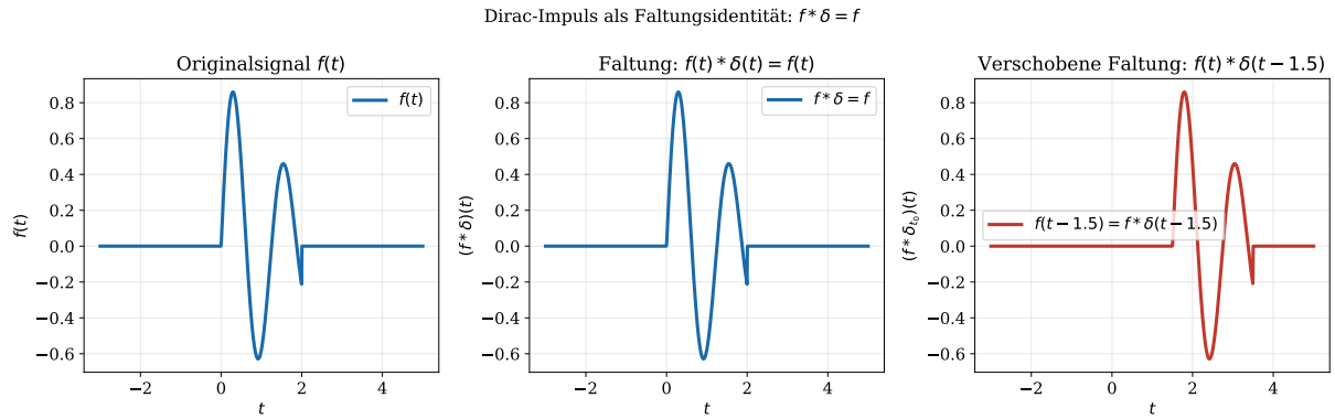
Figure 7: Dirac als neutrales Element der Faltung. Links: Originalsignal f(t) . Mitte: f * \delta = f (keine Veränderung). Rechts: f * \delta_{t_0} verschiebt das Signal um t_0 = 1.5 nach rechts.
