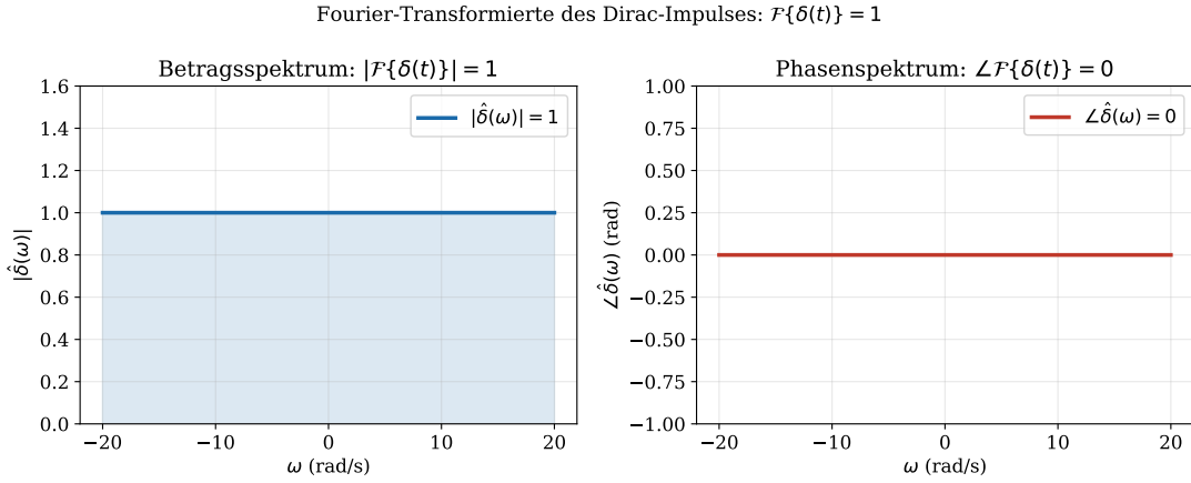
Figure 4: Fourier-Transformierte des Dirac-Impulses: das Betragsspektrum ist konstant 1 (weißes Rauschen / weißes Spektrum), und die Phase ist identisch 0. Dies bedeutet, dass der Dirac-Impuls alle Frequenzen mit gleicher Amplitude enthält.
