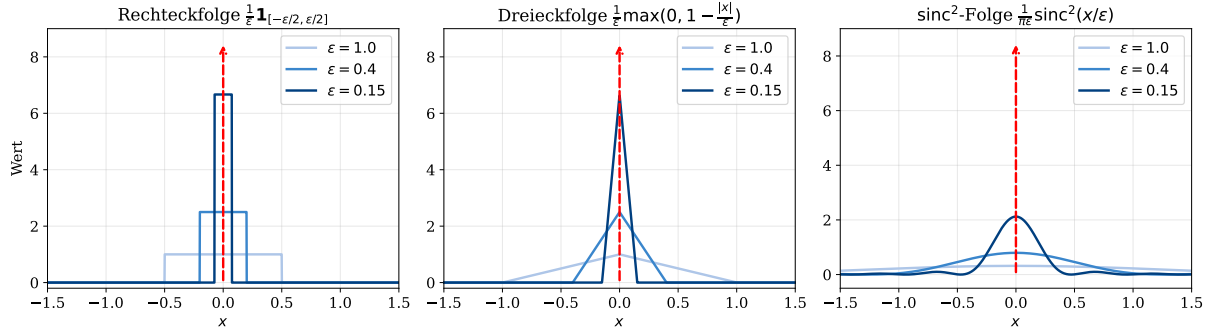
Figure 5: Drei verschiedene Näherungsfolgen für den Dirac-Impuls bei \varepsilon \in \{1.0, 0.4, 0.15\} : Rechteckfolge (links), Dreieckfolge (Mitte) und Sinc 2 -Folge (rechts). In allen Fällen schrumpft die Breite proportional zu \varepsilon , während die Höhe um 1/\varepsilon wächst, sodass die Fläche konstant 1 bleibt. Der rote Pfeil symbolisiert den Grenzwert \delta(t) .
