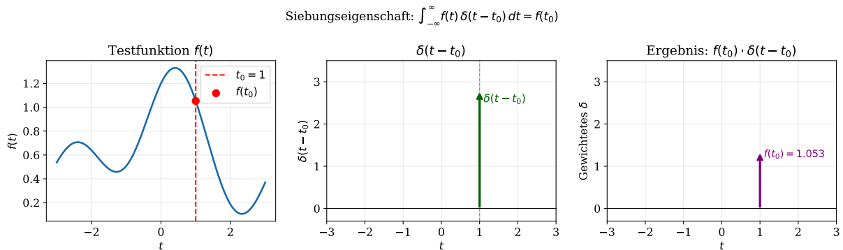
Figure 2: Illustration der Siebungseigenschaft. Links: die Testfunktion f(t) . Mitte: der verschobene Dirac-Impuls \delta(t - t_0) bei t_0 = 1 . Rechts: Das Produkt f(t) \cdot \delta(t - t_0) liefert nach Integration genau den Funktionswert f(t_0) .
