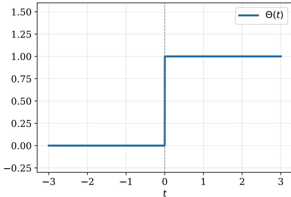
Heaviside-Stufenfunktion \Theta(t)
