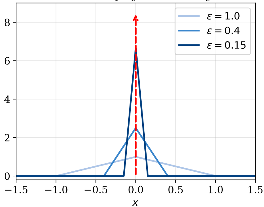
Dreieckfolge \frac{1}{\varepsilon} \max(0, 1 - \frac{|x|}{\varepsilon})
