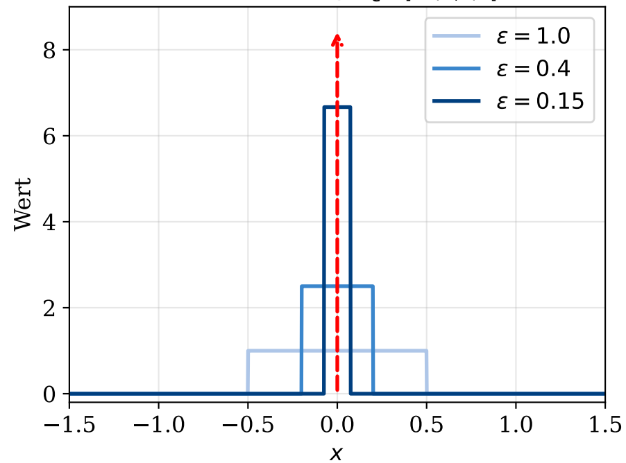
Rechteckfolge \frac{1}{\varepsilon} \mathbf{1}_{[-\varepsilon/2, \varepsilon/2]}
