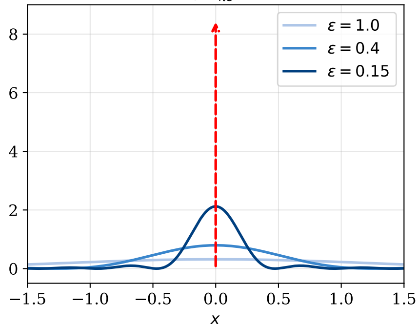
\text{sinc}^2 -Folge \frac{1}{\pi\varepsilon} \text{sinc}^2(x/\varepsilon)
