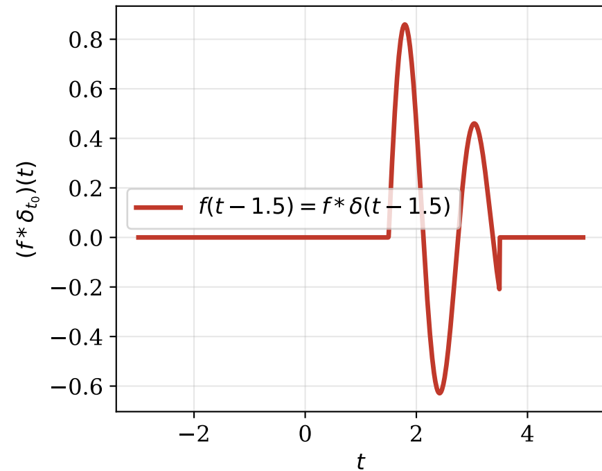
Verschobene Faltung: f(t) * \delta(t - 1.5)
