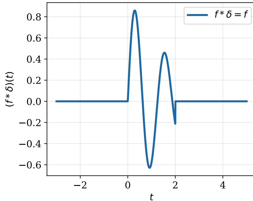
Faltung: f(t) * \delta(t) = f(t)
