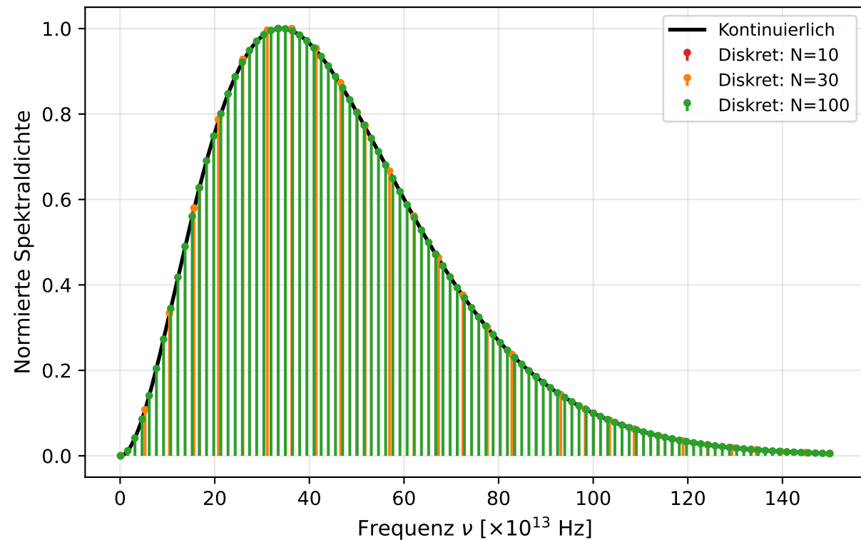
Kontinuum vs. diskrete Moden
