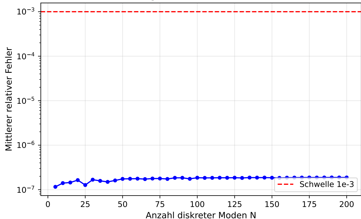
Konvergenz: Diskret => Kontinuum
