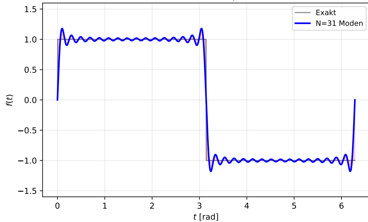
N = 31 harmonische Oberwellen | RMS-Fehler = 0.1126
