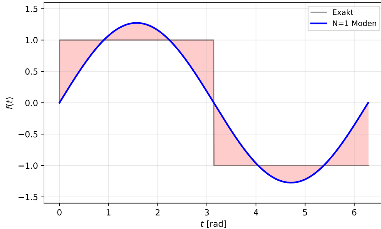
N = 1 harmonische Oberwellen | RMS-Fehler = 0.4350
