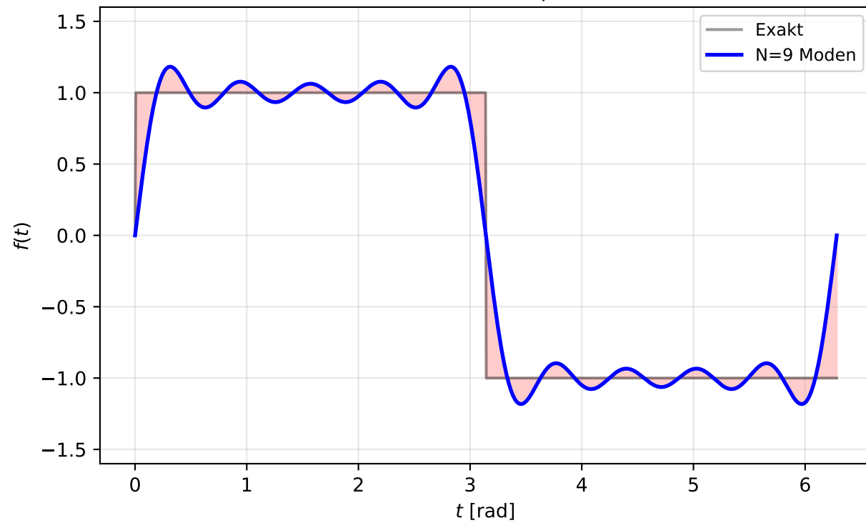
N = 9 harmonische Oberwellen | RMS-Fehler = 0.2009
