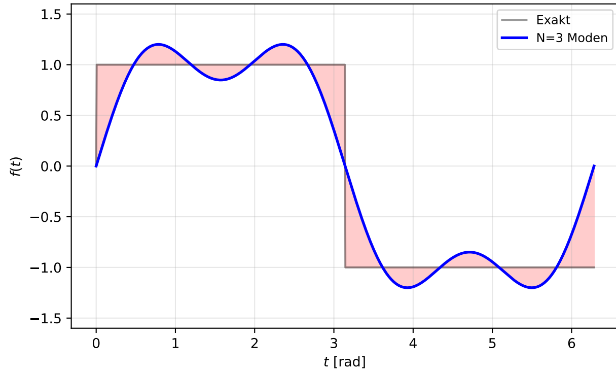
N = 3 harmonische Oberwellen | RMS-Fehler = 0.3151
