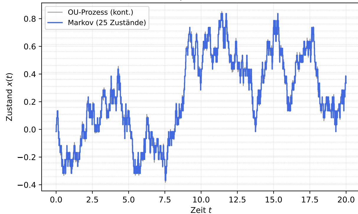
25 Zustände | RMS-Fehler = 0.0145
