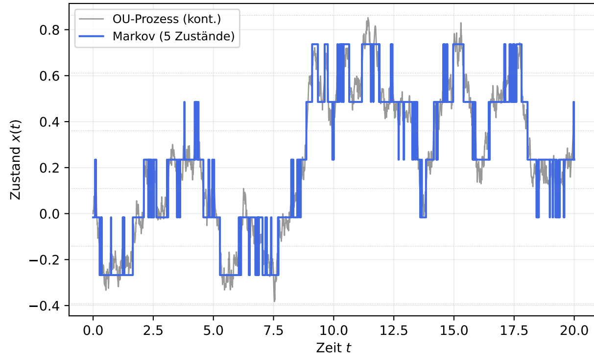
5 Zustände | RMS-Fehler = 0.0718
