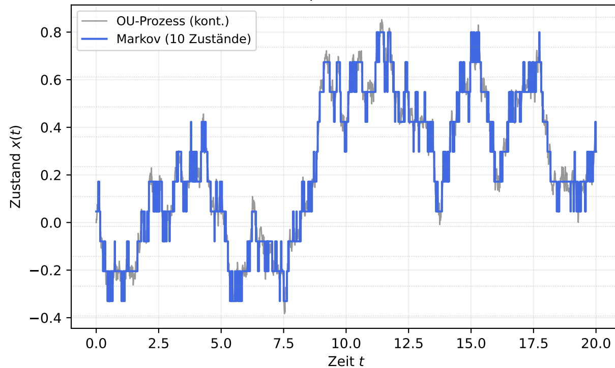
10 Zustände | RMS-Fehler = 0.0362
