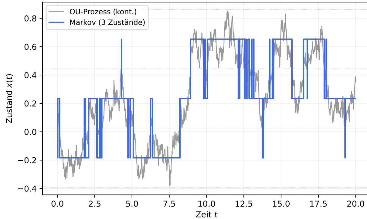
3 Zustände | RMS-Fehler = 0.1134
