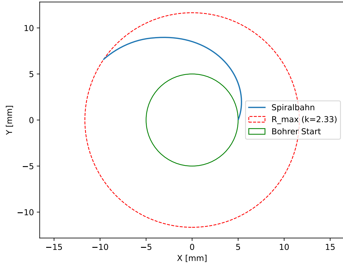
Spiralbahn (Material Typ 1)
