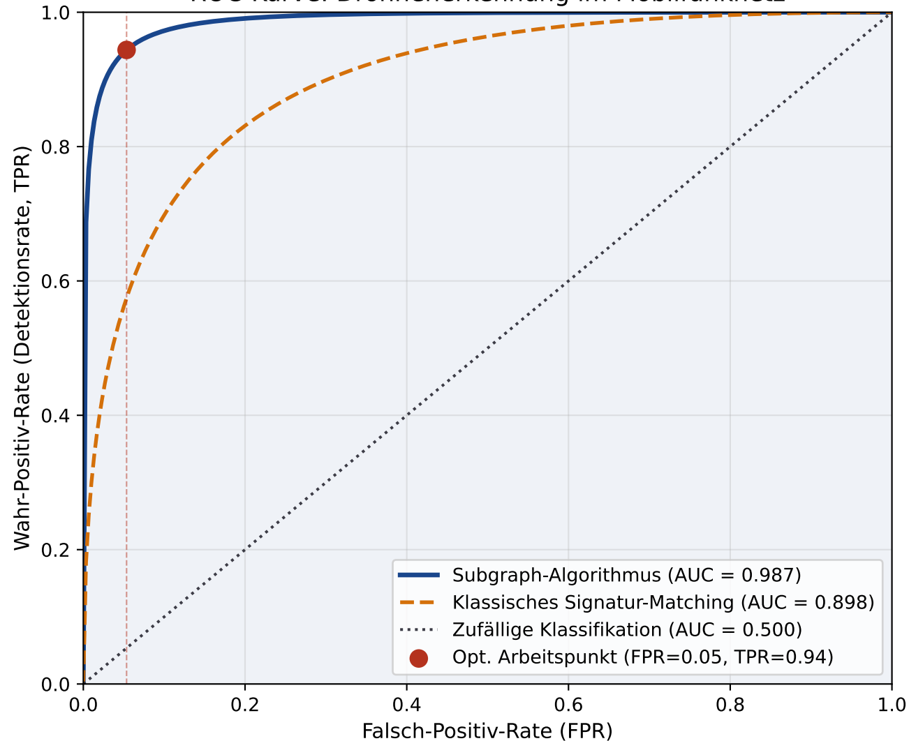
ROC-Kurve: Drohnenerkennung im Mobilfunknetz
