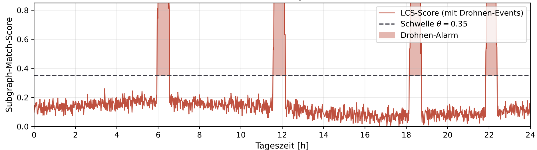
Mit simulierten Drohnen-Einflügen (Echtzeit-Detektion)
