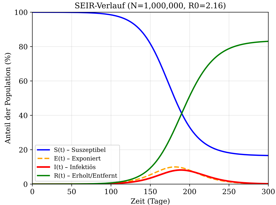
Abbildung 1: SEIR-Modell - Ebolavirus-Infektionsdynamik
