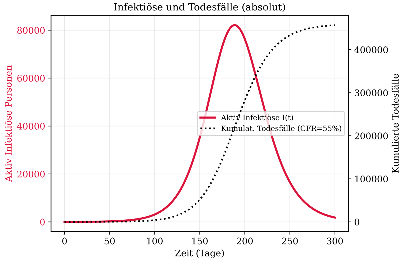
Abbildung 1: SEIR-Modell - Ebolavirus-Infektionsdynamik
