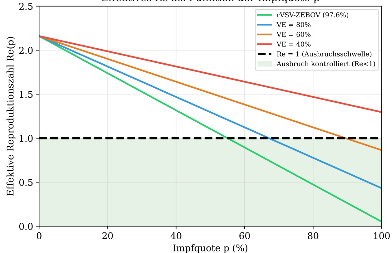
Effektives R_e als Funktion der Impfquote p
