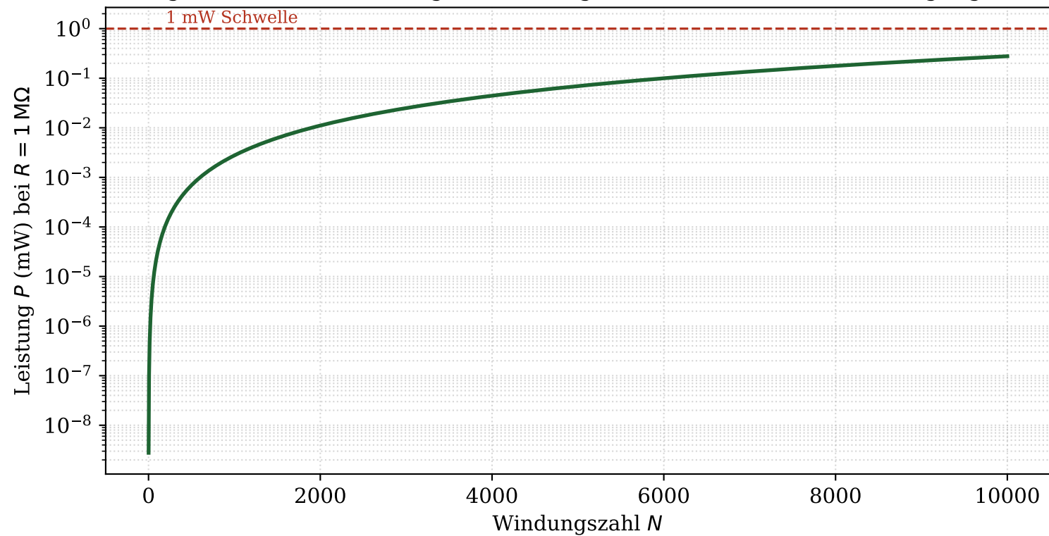
Abgeschätzte Nutzleistung vs. Windungszahl ( A = 1 \text{ km}^2 , Sturmbedingungen)
