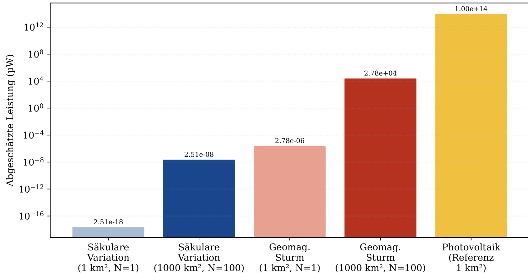
Vergleich induzierter Leistungen - verschiedene Szenarien
