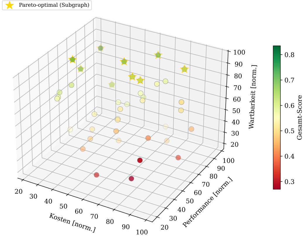
Figure 9: 3D-Entwurfsraum für 40 Entwurfsalternativen in den Dimensionen Kosten, Performance, Wartbarkeit. Die Farbe kodiert den normierten Gesamt-Score. Goldene Sterne markieren die durch den Subgraph-Algorithmus identifizierten Pareto-optimalen Entwürfe.
