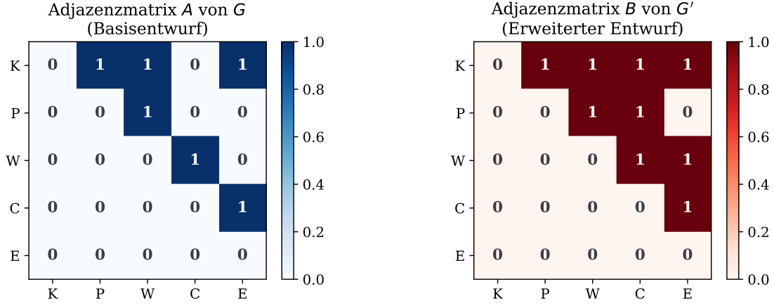
Figure 4: Adjazenzmatrizen A (Entwurf G ) und B (Entwurf G' ). Alle Einträge A_{ij} = 1 sind auch in B enthalten ( A \subseteq B ), was die Subgraph-Beziehung G \subseteq G' formell bestätigt. Zeilenbeschriftung: K=Kosten, P=Performance, W=Wartbarkeit, C=Konfigurierbarkeit, E=Erreichbarkeit.
