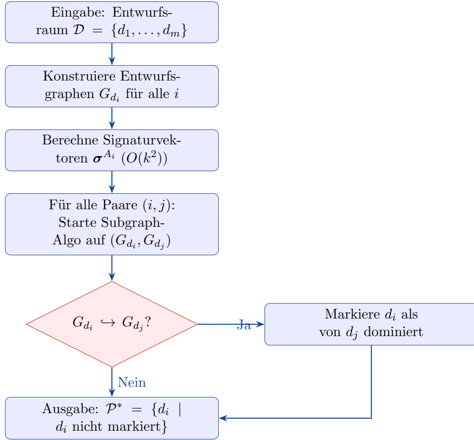
Figure 6: Ablaufdiagramm des Gesamtalgorithmus zur Pareto-Front-Bestimmung mittels Subgraph-Isomorphismus. Für jedes Paar (d_i, d_j) wird der Subgraph-Algorithmus [1] mit \Theta(k^3) aufgerufen.
