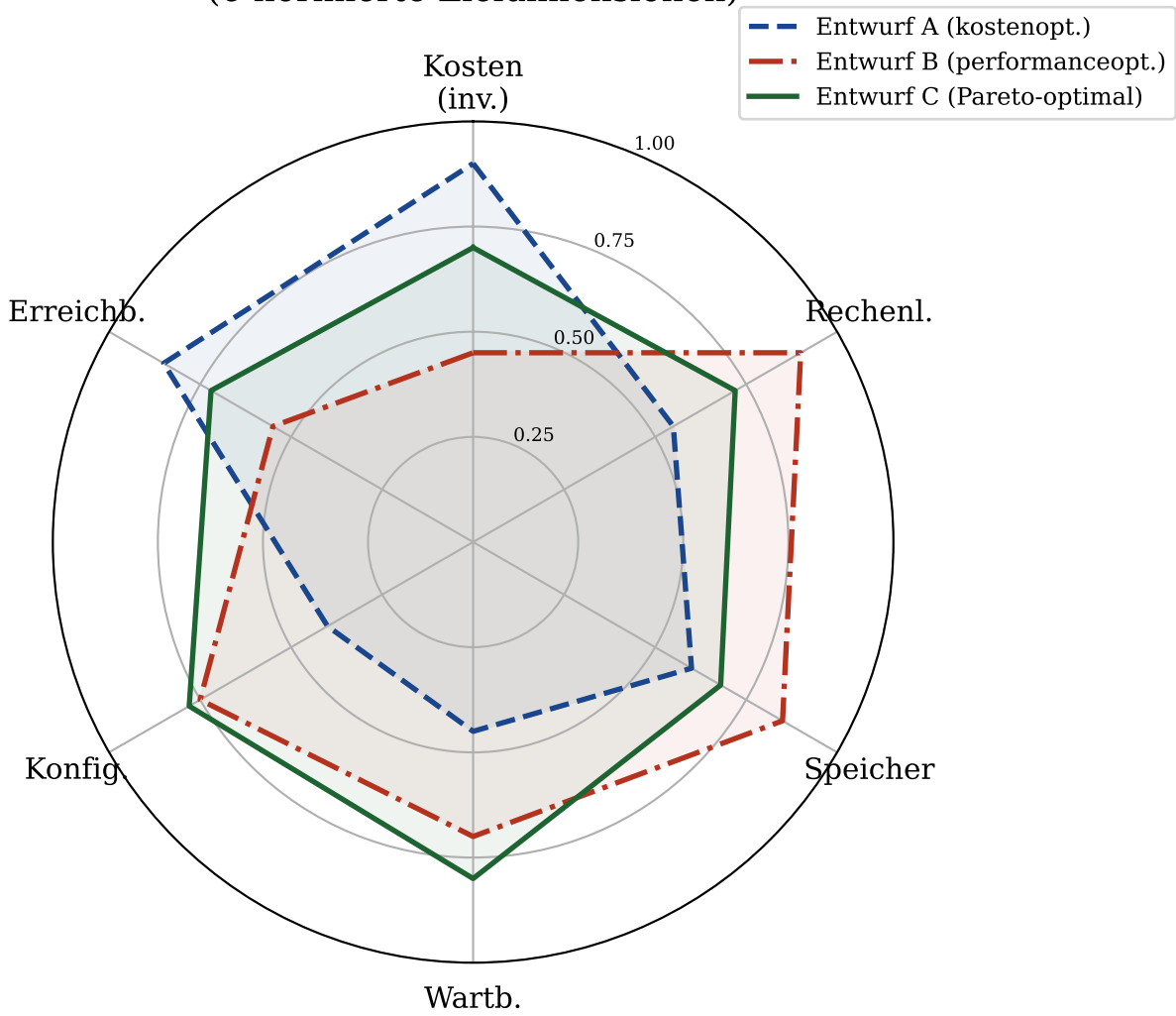
Abb. 2 – Multi-Kriterien-Radar für Embedded-Systems-Entwurf (6 normierte Zieldimensionen)
