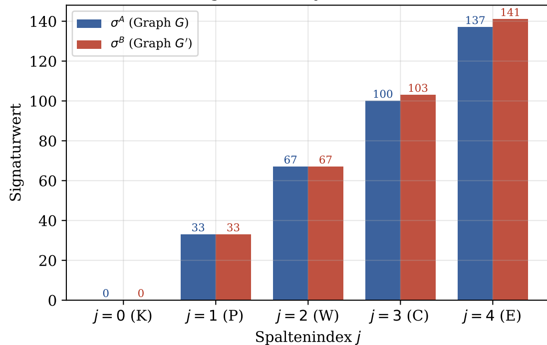
Signatur-Arrays \sigma^A und \sigma^B
