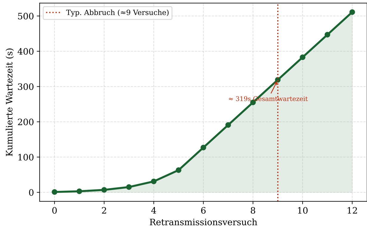
Kumulierte Wartezeit bis Verbindungsabbruch (TCP RTO, RFC 6298)
