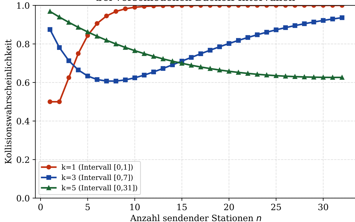
CSMA/CD: Kollisionswahrscheinlichkeit bei verschiedenen Backoff-Intervallen
