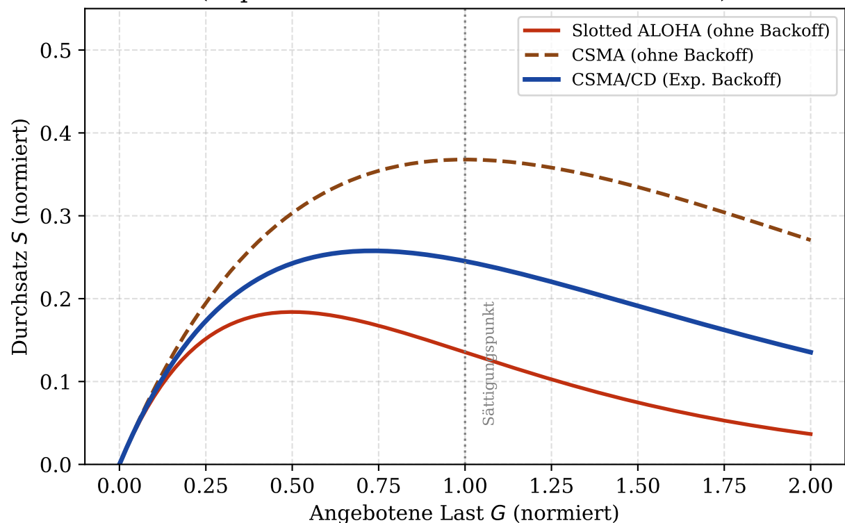
Netzwerkdurchsatz vs. angebotene Last (Exponential Backoff verbessert Stabilität)
