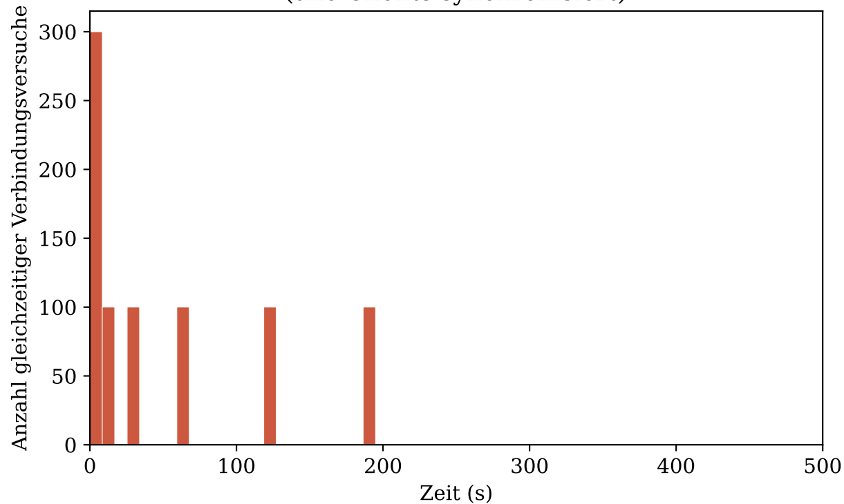
Ohne Jitter: Thundering Herd (alle Clients synchronisiert)
