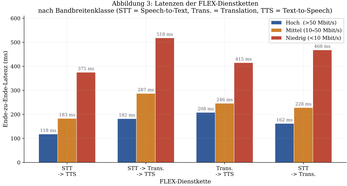
Figure 3: Ende-zu-Ende-Latenzen der FLEX-Dienstketten. Die dreistufige Kette STT→Translate→TTS erreicht bei Niedrigbandbreite 518ms, was durch bandbreitenklassenbasiertes Routing auf leichtgewichtigeren Einzeldiensten in solchen Regionen kompensiert wird.
