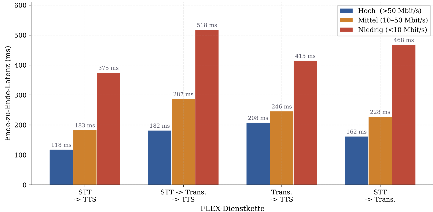
Abbildung 3: Latenzen der FLEX-Dienstketten nach Bandbreitenklasse (STT = Speech-to-Text, Trans. = Translation, TTS = Text-to-Speech)
