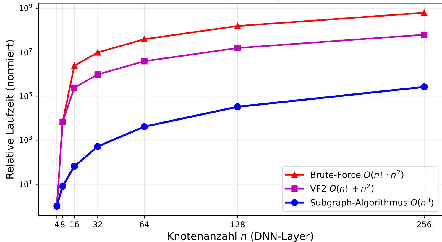
Laufzeitvergleich: Subgraph-Algorithmus vs. klassische Ansätze für DNN-Topologie-Matching auf FPGA
