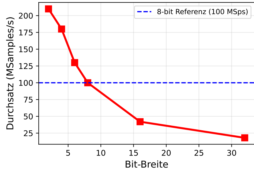
Inferenzdurchsatz nach Quantisierungstiefe
