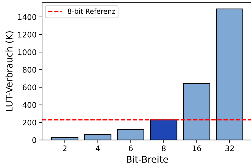
LUT-Ressourcenverbrauch nach Quantisierungstiefe
