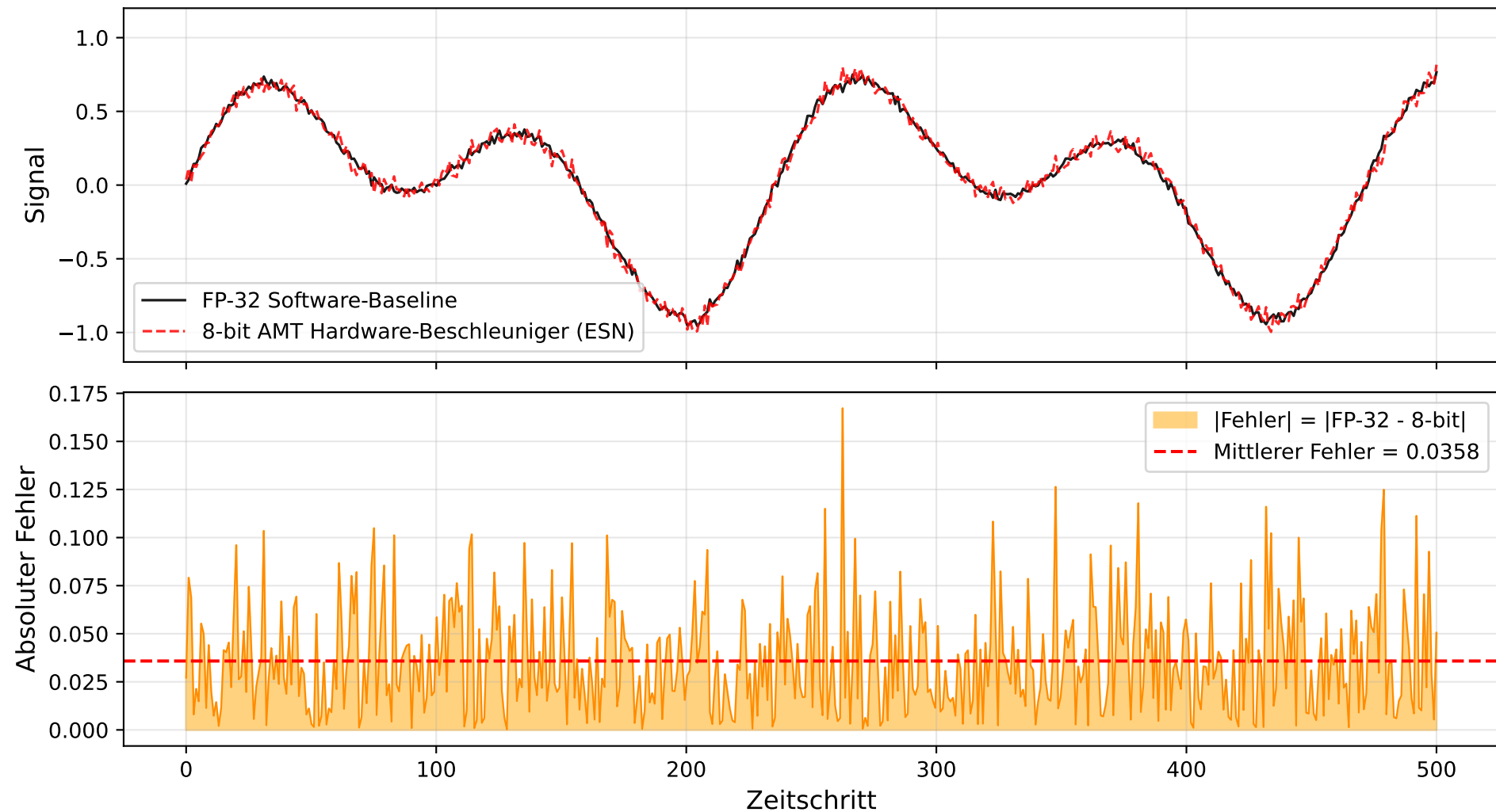
Mackey-Glass Vorhersage: FP-32 vs. 8-bit quantisierter ESN-FPGA-Beschleuniger (500 Zeitschritte)
