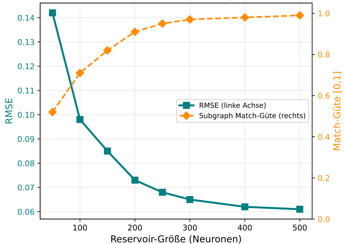
RMSE und Subgraph-Match-Güte bei ESN-FPGA-Optimierung
