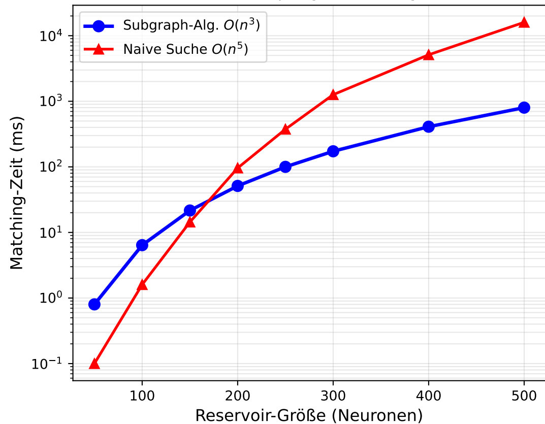
Subgraph-Matching-Laufzeit bei ESN-Topologie-Erkennung
