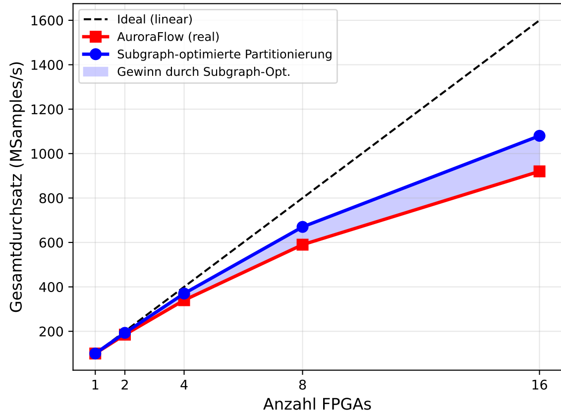
Multi-FPGA Skalierung: Subgraph-Optimierung vs. Standard-AuroraFlow
