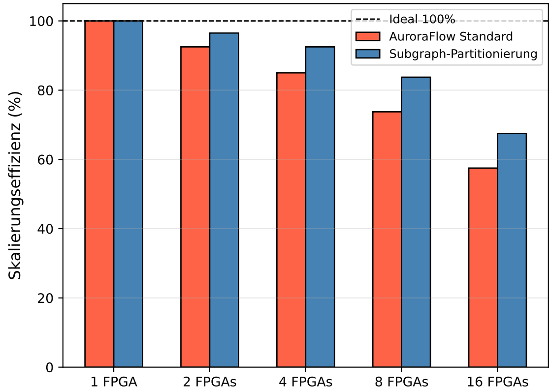
Skalierungseffizienz bei Multi-FPGA-Deployment
