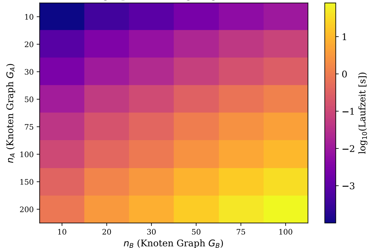
Laufzeit-Heatmap T(n_A, n_B) Subgraph-Matching ( \log_{10} -Skala)
