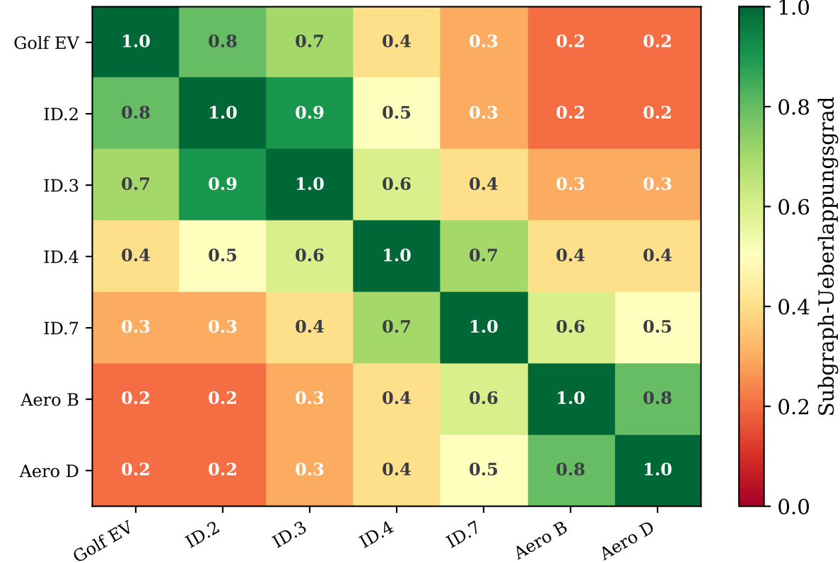
Subgraph-Überlappungsmatrix für alle VW EV-Plattformmodelle
