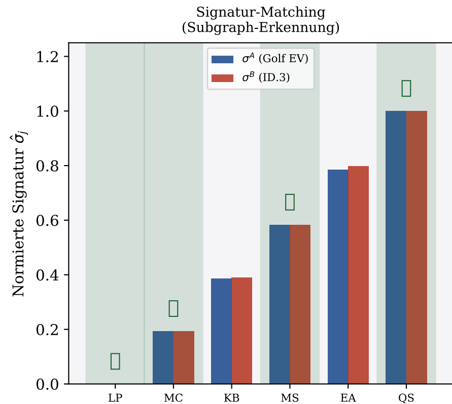
Abb. 2 – Subgraph-Signatur-Matching zweier Elektrofahrzeug-Produktionsvarianten (grüne Markierung = übereinstimmende Prozessmodule → erkannter Subgraph)
