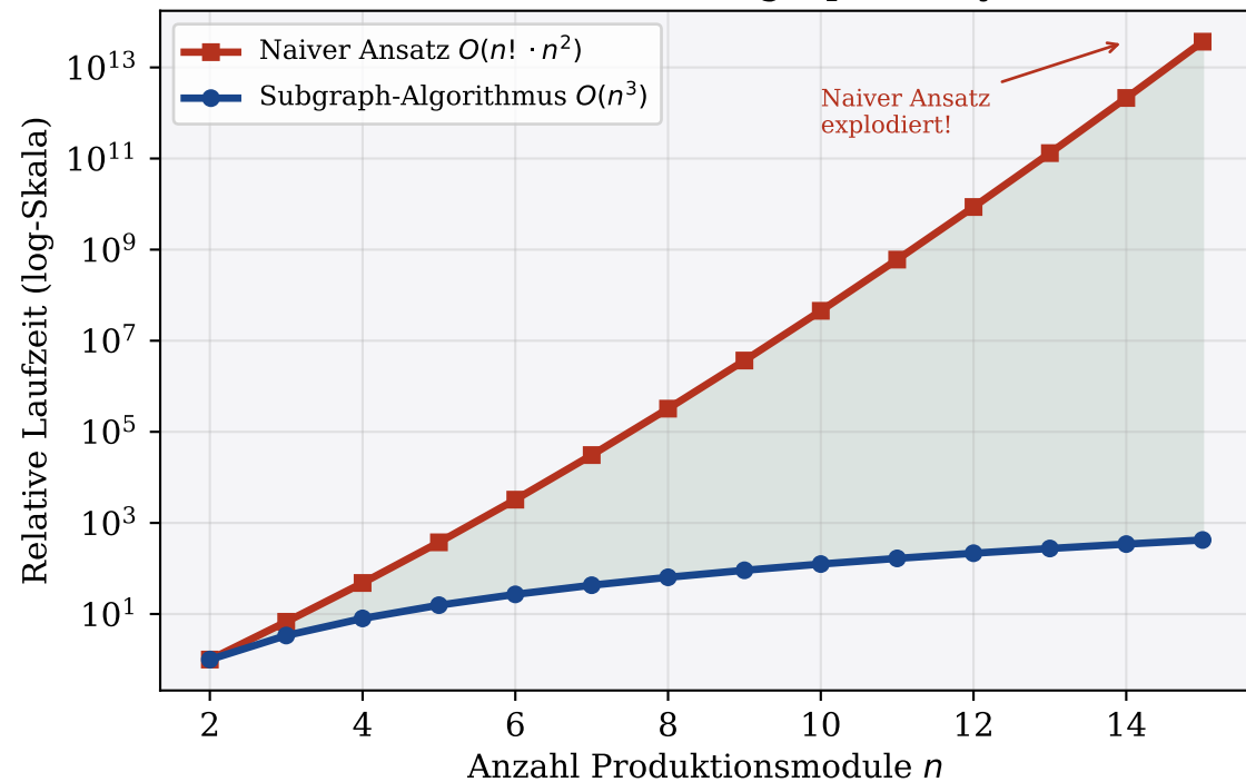
Laufzeitvergleich: Naiv vs. Subgraph bei der Produktionsgraph-Analyse
