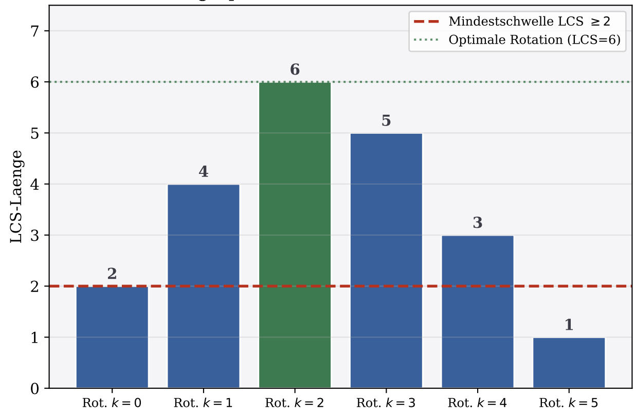
LCS-Laenge je zyklischer Rotation (Subgraph-Match zweier Prozessketten)
