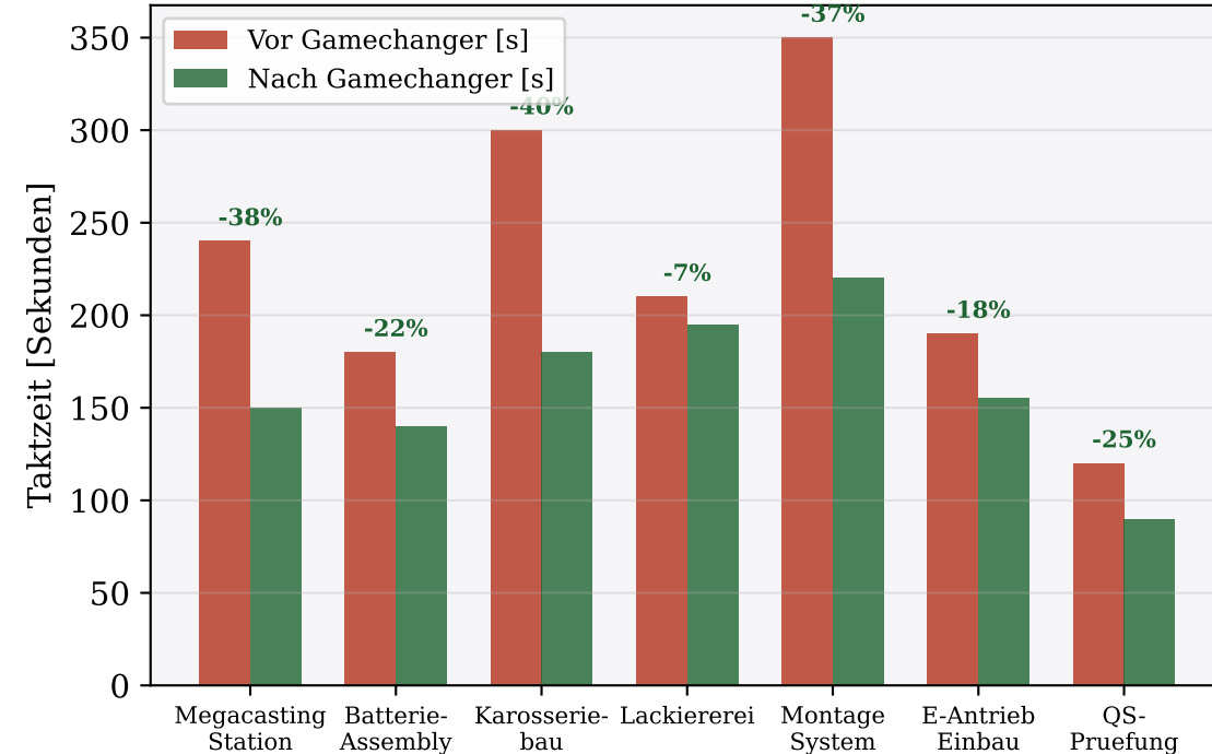
Taktzeit-Optimierung je Station durch Subgraph-basiertes Scheduling
