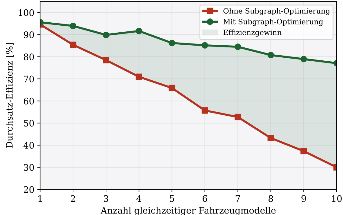
Produktionsdurchsatz vs. Modellvarianten-Anzahl
