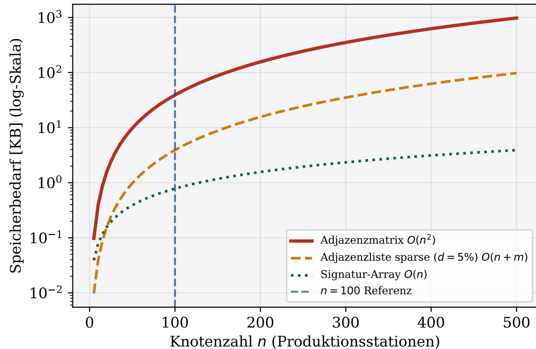
Speicherkomplexität verschiedener Graphrepräsentationen
