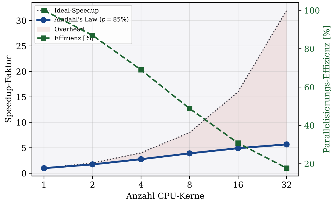
Parallelisierbarkeit der Rotations- berechnungen (Amdahlsches Gesetz)
