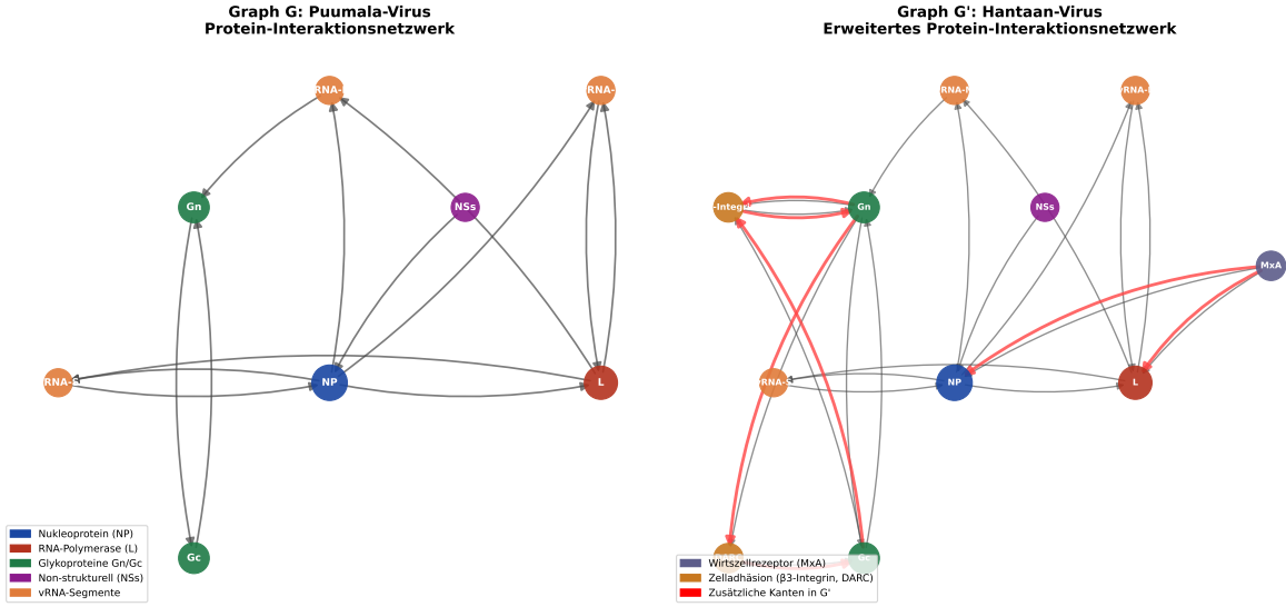
Figure 2: Links: Graph G (Puumala-VPIN). Rechts: Graph G' (Hantaan-VPIN als Supergraph). Zusätzliche Kanten in G' \setminus G sind rot markiert.
