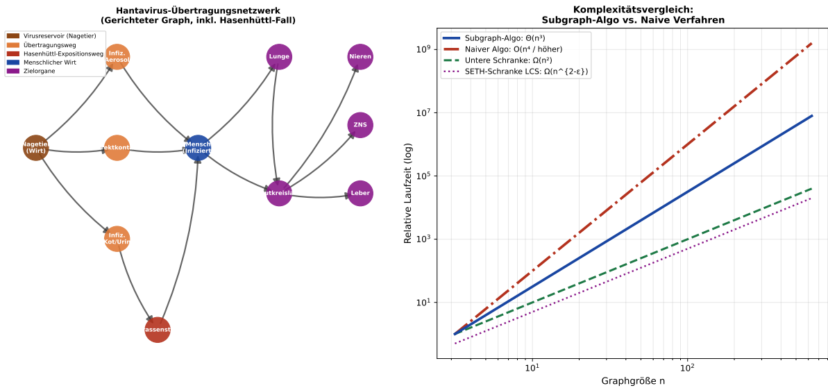
Figure 6: Links: Virales Übertragungsnetzwerk (Hasenhüttl-Expositionsweg rot). Rechts: Logarithmischer Komplexitätsvergleich.
