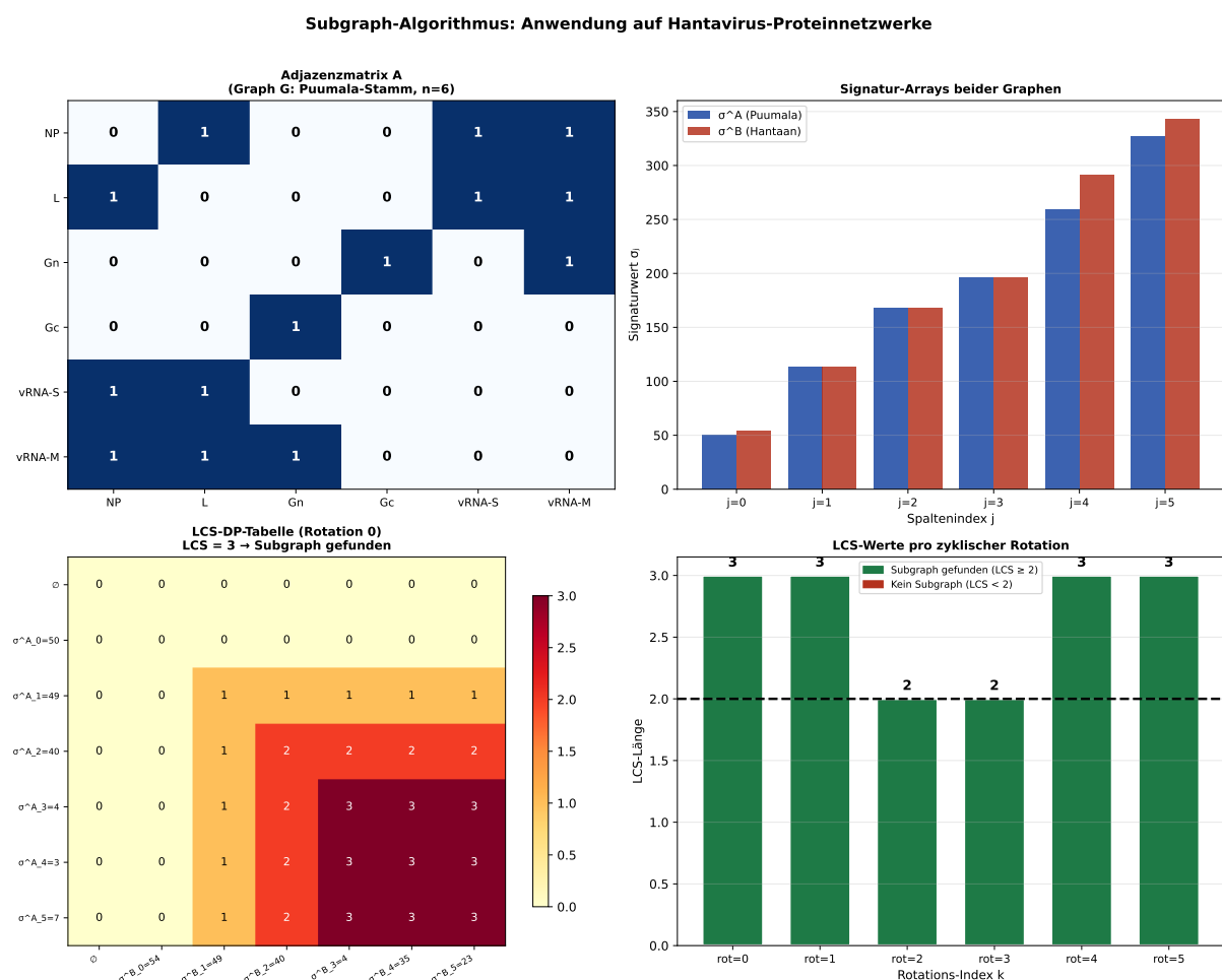
Figure 3: Vollständige Algorithmusanwendung: Adjazenzmatrix, Signaturvergleich, LCS-DP-Tabelle und Rotationsanalyse für PUUV vs. HTNV.
