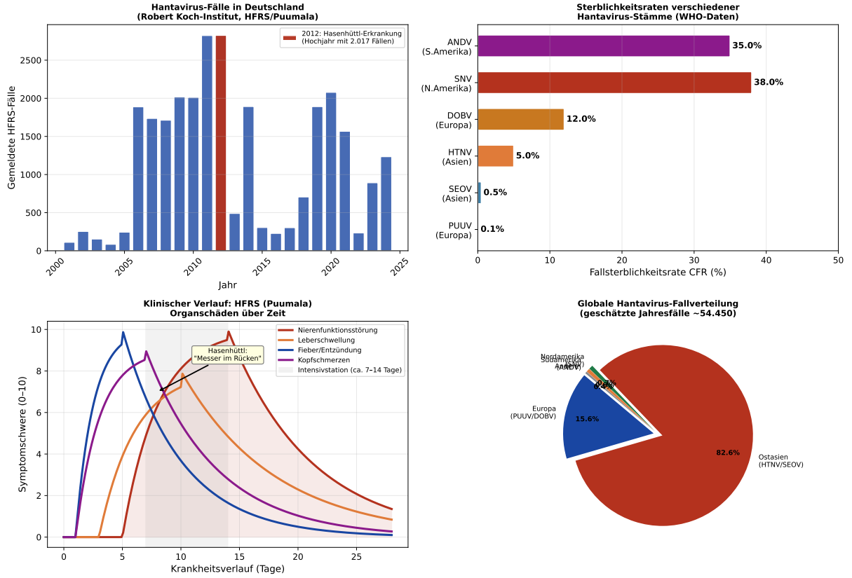
Figure 4: Epidemiologische Übersicht: Fallzahlen Deutschland (mit Markierung 2012), CFR-Vergleich, klinischer Verlauf, globale Verteilung.
