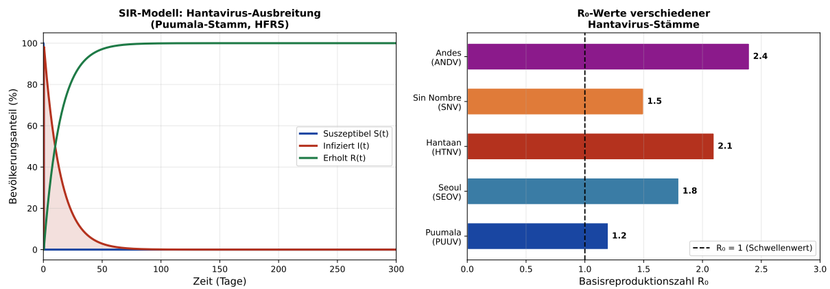
Figure 1: Links: SIR-Modell der Hantavirus-Ausbreitung (Puumala-Stamm). Rechts: Basisreproduktionszahlen R_0 verschiedener Hantavirus-Stämme. Der Schwellenwert R_0 = 1 (gestrichelte Linie) trennt Ausbruchs- von Abdampfsituationen.
