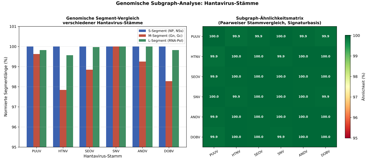
Figure 5: Links: Normierte genomische Segmentlängen der sechs Hauptstämme. Rechts: Subgraph-Ähnlichkeitsmatrix (Signatur-basiert, Kosinus-Distanz).
