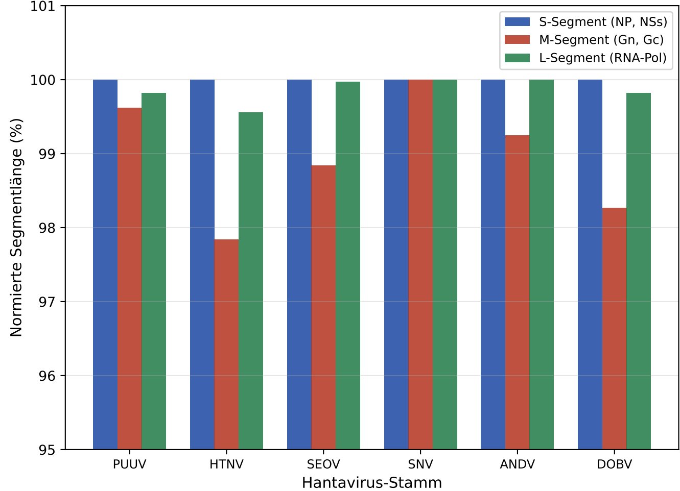
Genomische Segment-Vergleich verschiedener Hantavirus-Stämme
